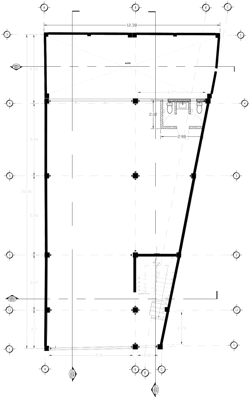
PLANTA NIVEL 2
